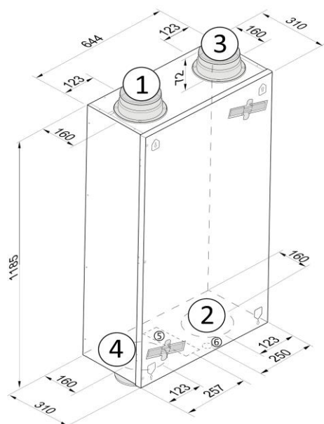
RENOVENT SKY 300
